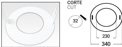
ACCESORIO CIRCULAR PARA TECHO DE PLADUR CIRCULAR FRAME RECESSED MOUNTING
