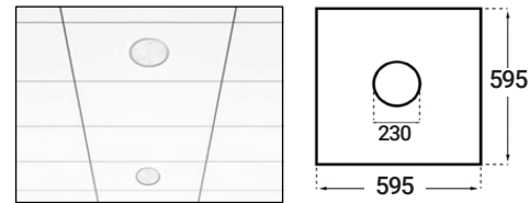
ACCESORIO CUADRADO PARA TECHO DE PERFLERIA VISTA SQUARE FRAME RECESSED MOUNTING
